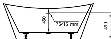
SEÇÃO AA
