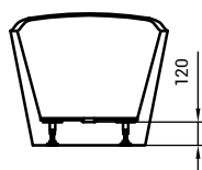
SEÇÃO BB
